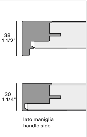
sezione anta - door section
