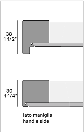
sezione anta - door section
