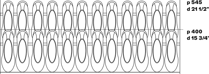
larghezza mm 1263 width 49 3/4"
